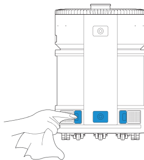
Capteurs de signal du pare-chocs anticollision et de la station de charge
